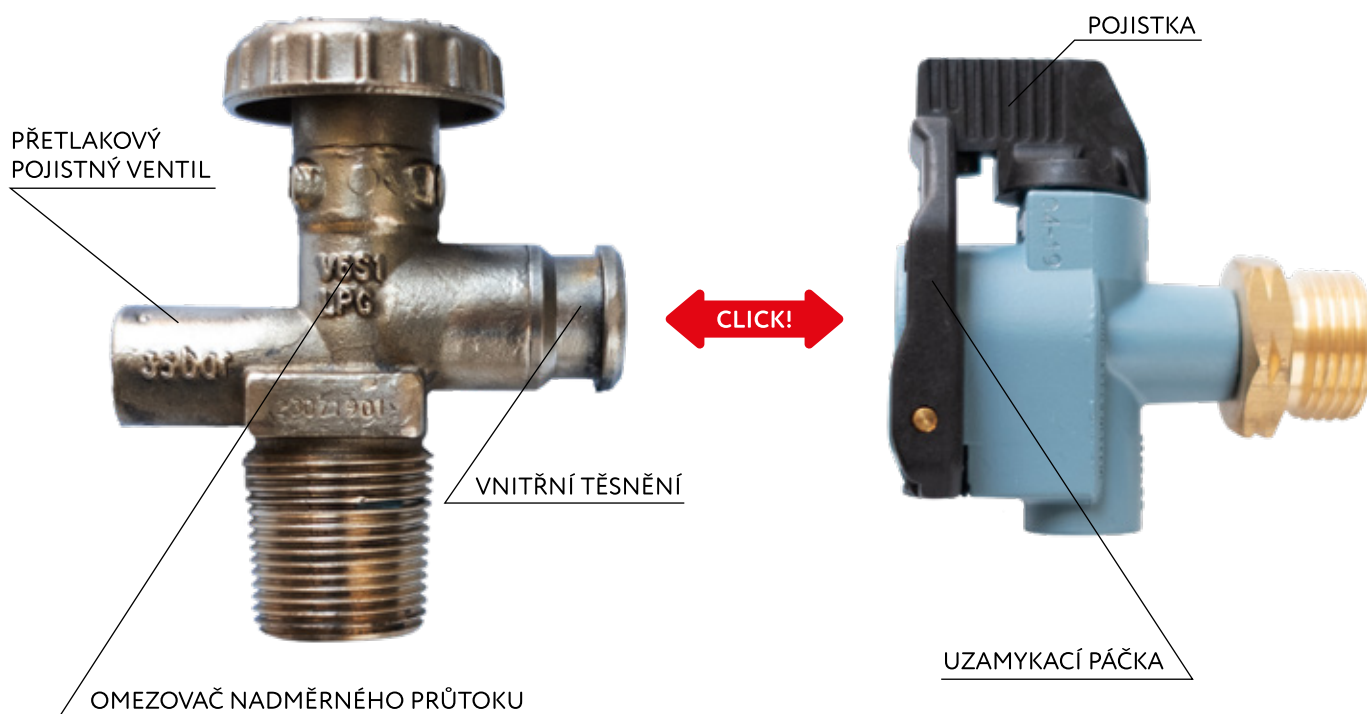
BEZPEČNOSTNÍ VENTIL
